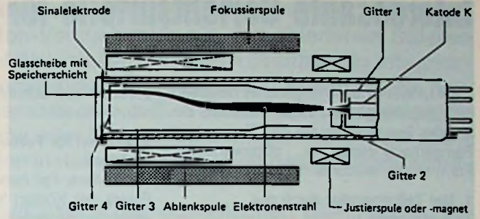
Bild 4: Schematischer Aufbau eines Vidikons ▲
