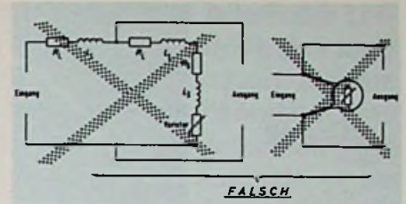
Bild 1: So sind Varistoren wenig wirksam
