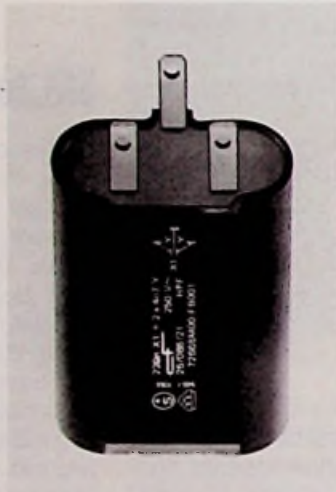
Bild 1: Überspannungssichere Funkentstörkombination (Condens. Fribourg-Pressbild)
