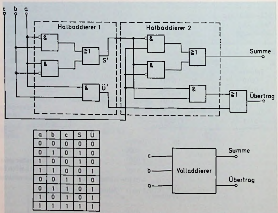
Bild 4.3.2: Zusammenwirken zweier Halbaddierere zu einem Volladdierer
