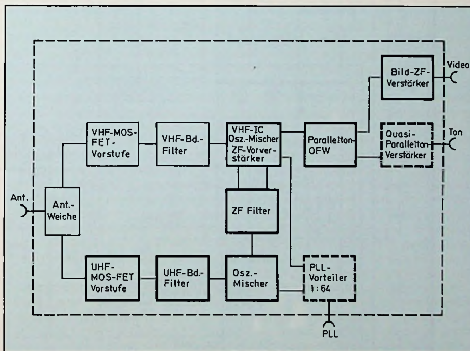
Bild 1: HF-ZF-Modul-Schaltungskonzept
