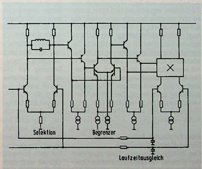
Bild 5: Innere Schaltungsstruktur des Quasi-Parallelton-Demodulators
