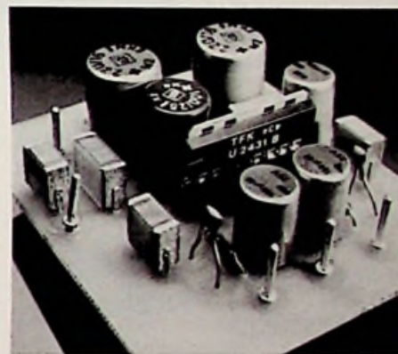
Bild 7: Integrierte Schaltung mit ihren Peripherie-Elementen für einen Stereo-Verstärker mit 1 W je Kanal (Telefunken-electronic-Pressbild)
